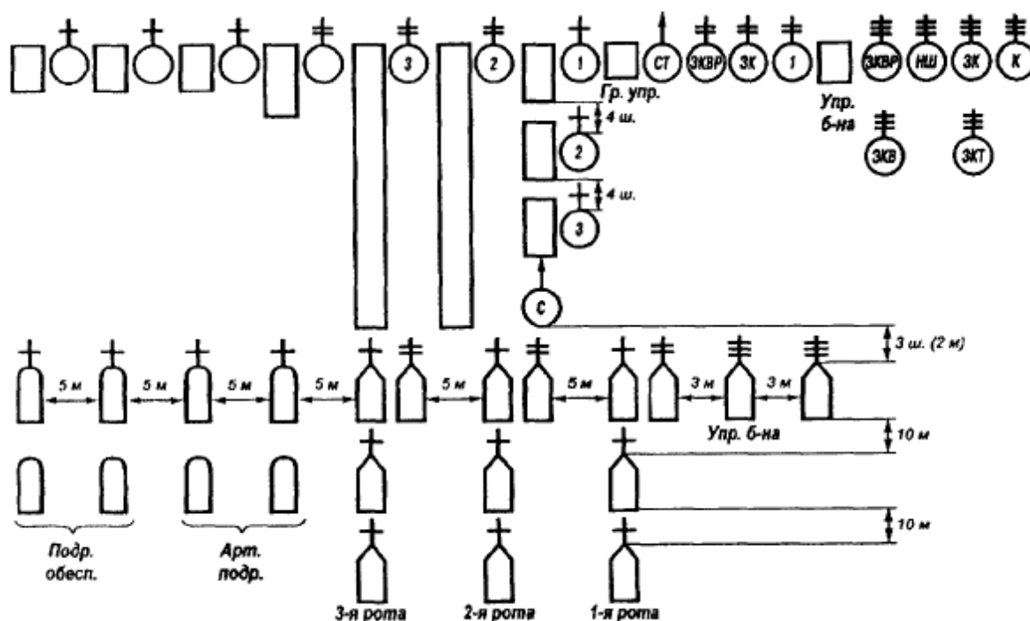
Рис.37. Построение роты с личным составом впереди машин: личный состав и машины - в линию взводных колонн
